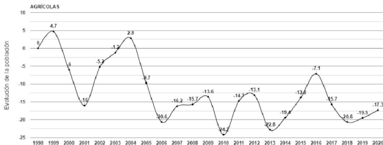
Gráfica 57. Evolución del índice de las aves asociadas a medios agrícolas arbóreos en Castilla-la Mancha.
