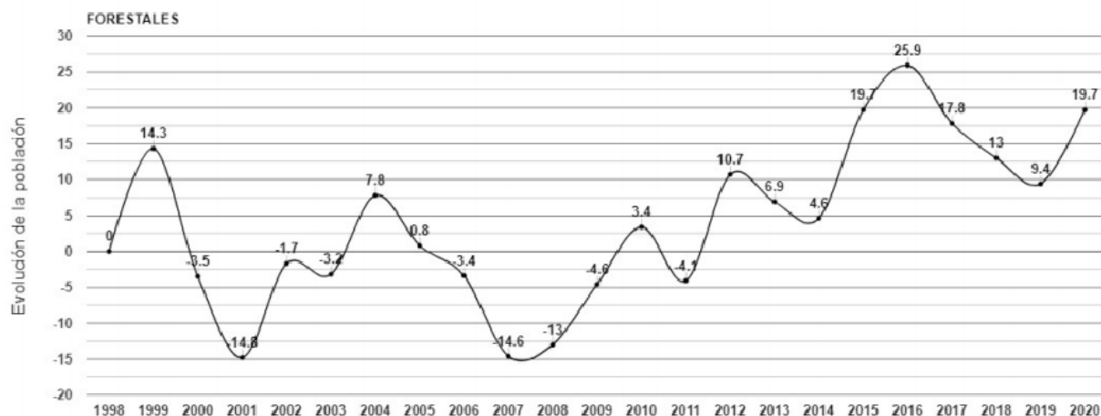
Gráfica 59. Evolución del índice de las aves asociadas a medios forestales.
